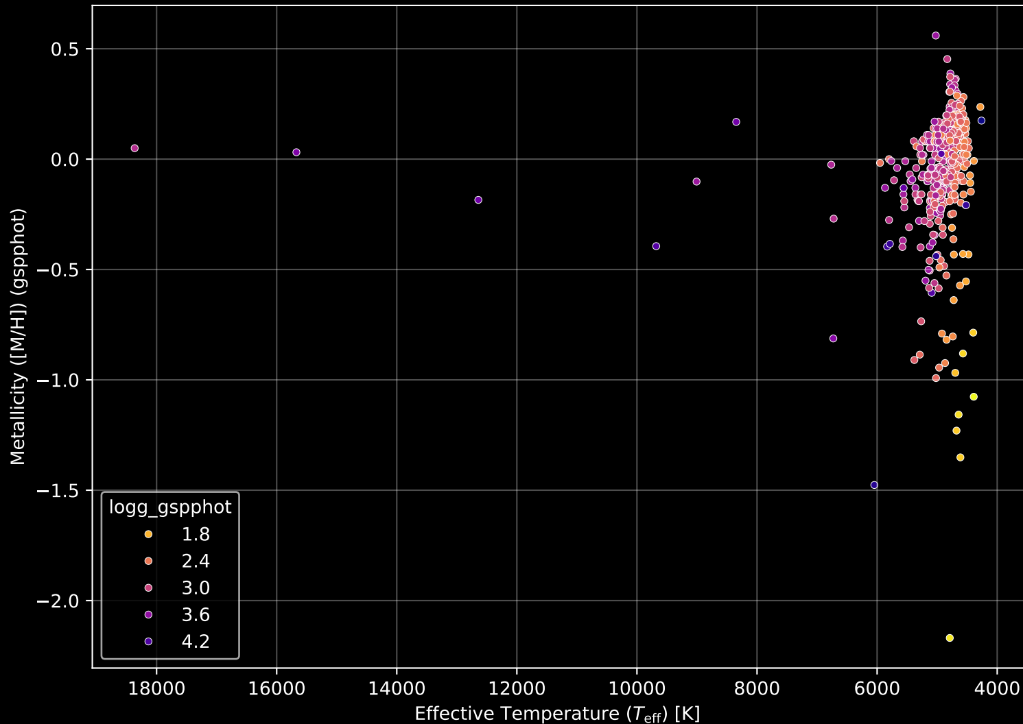
APOGEE DR17 Field: [300-04] Stellar Population Parameters (n= 475)
